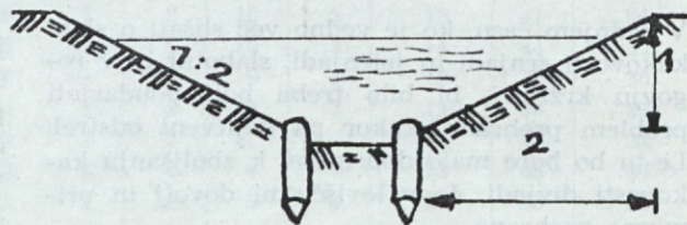
Prerez jarka v pešeni zemlji z utrjenim dnom
