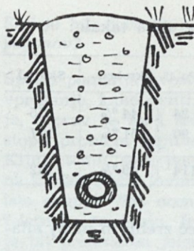
Drenažni jarek s posebno drenažno cevjo
