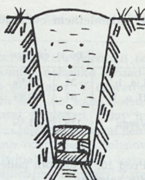
Drenažni jarek s cevjo iz zložene opeke
