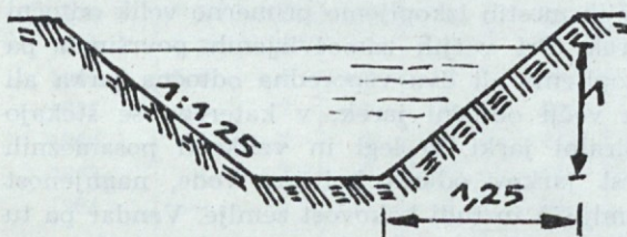
Prerez jarka v ilovnati zemlji
