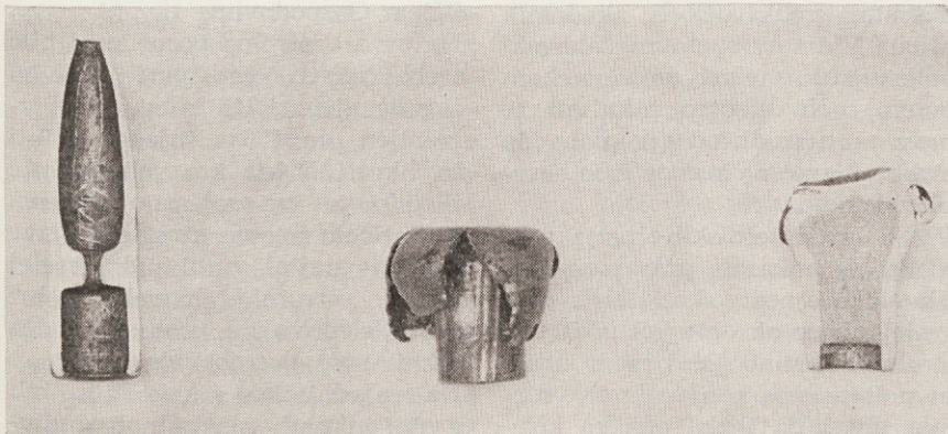
Slika 3: Levo predeljena krogla Nosler, v sredi njena »gobica«. Kratke zastavice dokazujejo zmaličenje po sl. 2. Desno prerezana popravljená Nosler, po strelu se je nabuhnila (ABC — varianta I).
