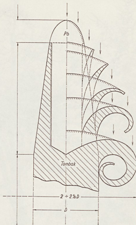
Slika 4: Potek zmaličenja pri novi krogli: končna oblika je ostrorobna rozeta z vase zasukanimi zastavicami (»ovnovi rogovi«), ki se trdno naslonijo na razmeroma dolg valjasti vodilni del krogle. Podobna je »kronskemu rezkarju«.
