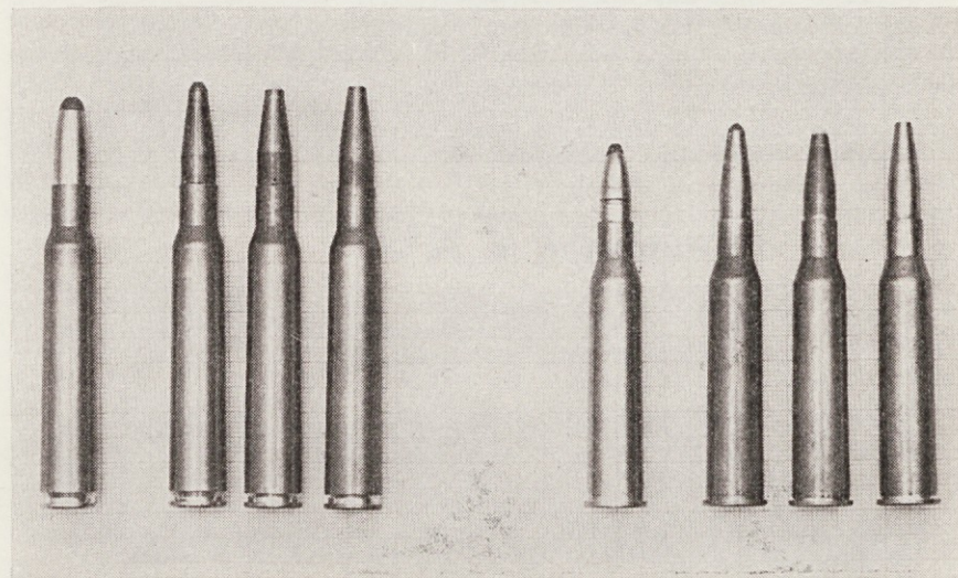
Slika 7: Levo — trije naboji HP-7 \times 64 ABC: svinčeni vložek 10,6 g, plastični vložek (vrh slabše viden, ker je bel) in odrezana konica. Zraven za primerjavo H P — TM (delni plašč) 11 g Desno — trije naboji 6,5 \times 57 R — ABC: svinčeni vložek 9 g, plastični vložek (vrh slabše viden, ker je bel) in odrezana konica. Zraven za primerjavo DWM-SM (Starkmantel) 8 g
