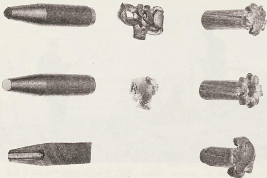
Slika 6: Zgoraj — krogla ABC s svinčnim vložkom, zraven nje ostanek takega vložka in taka krogla, le malo odprta, izstreljena skozi šibko divjad. Sredina — krogla ABC s plastičnim vložkom, zraven nje tak vložek po strelu in še ne povsem razprta krogla v obliki »kronskega rezkarja« (srnjad). Spodaj — ABC varianta III v prerezu brez svinca in ob njej običajna končna oblika po strelu skozi močno divjad, ustreza sl. 4, premer je večji od dveh kalibrov
