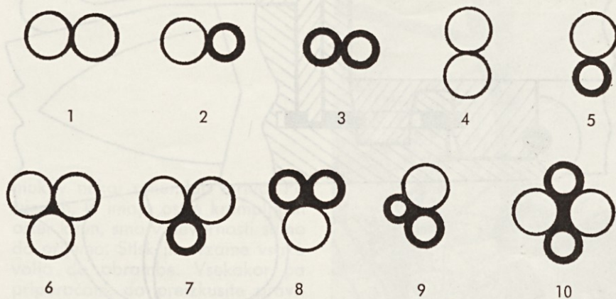
Skica 3. Možne namestitve cevi: 1 dvocevna šibrenica, 2 polrisanica, 3 dvocevna risanica, 4 bokarica šibrenica, 5 bokarica polrisanica, 6 trocevka šibrenica, 7 trocevka z risano cevjo, 8 trocevka z risanima cevema, 9 bokarica polrisanica s priveznjeno MK cevjo, 10 štiricevka, dve cevi za šibre, dve za kroglo
