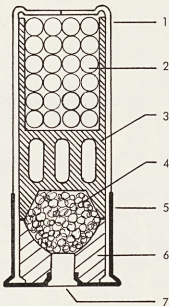
Skica 1. Sodoben šibreni naboj
