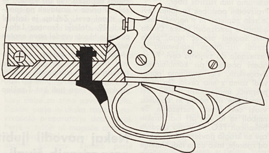
Skica 4. Lancaster zaklep pri petelinki
