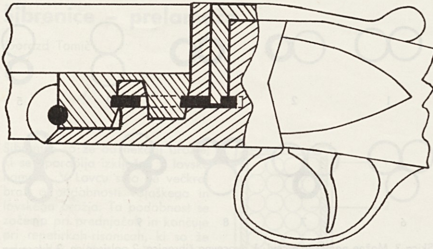
Skica 6. Dvojni klinasti zaklep pri bokarici; pri odpiranju se klin pomakne nazaj
