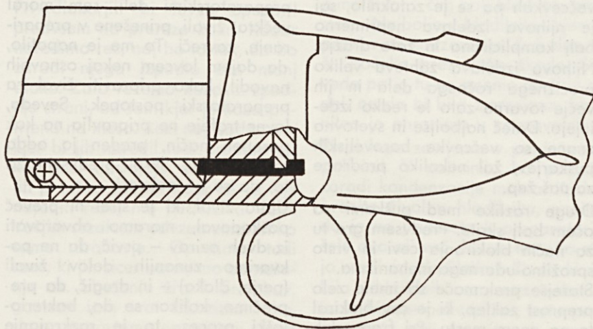
Skica 5. Enojni klinasti zaklep pri bokarici (klin počrtnjen)
