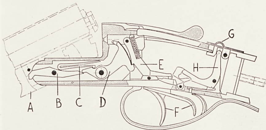
Skica 12. Sistem Anson & Deeley pri puški Crvena zastava M 64 in M 70: A – kopišček in cevi, B – vzvod za napenjanje petelinov, C – ploščata udarna vzmet, D – petelin z iglo v enem kosu, E – zatik petelina z vzmetjo, F – sprožilca, G – gumb varovalke, H – vzvod varovalke
