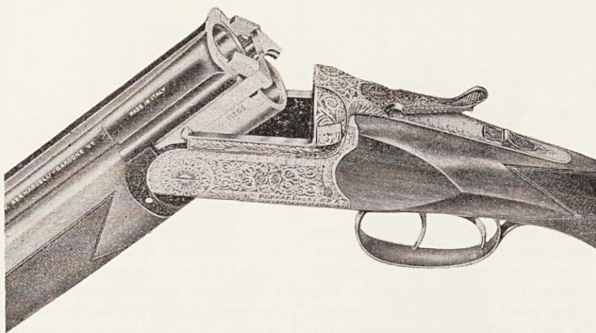
Skica 10. Dvojni Purdeyev zaklep pri bokarici Bernardelli Orione
