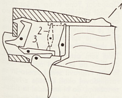
Skica 13. Varovalki. Prikazana varo- valka blokira sprožilec; črtkana blo- kira zatik petelina. Številke pomenijo: 1 – gumb varovalke, 2 – vzvod varo- valke, ki prepreči gib zatika, 3 – zatik petelina
