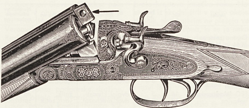
Skica 8. Greenerjev (enojni prečnozatični) zaklep. Pod cevema nastavek z izrezoma za dvojni klinasti zaklep
