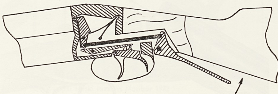
Skica 11. Starejša hamerles. S pritiskom na vzvod v smeri puščice se prek paličice (črna) napnejo notranji petlini.
