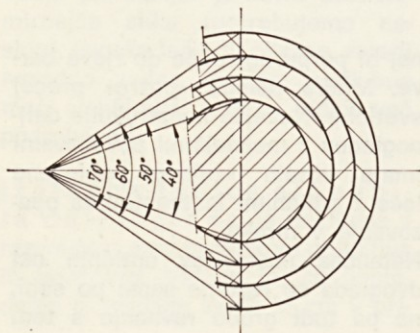
Primerjava površin zornega polja pri različnih navideznih zornih kotih
