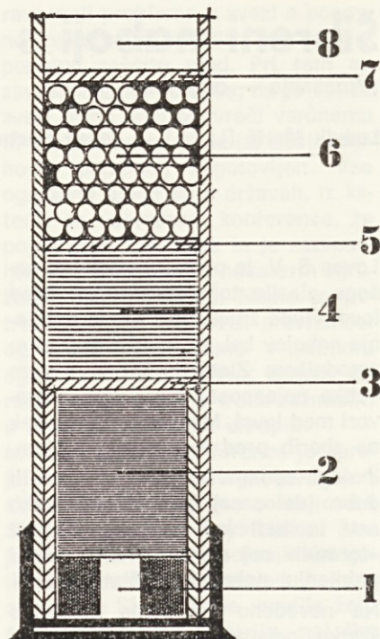
Prerez šibrenega naboja z vložkom: 1 — netilka, 2 — smodnik Zlatibor, 3 — poklopec nad smodnikom, 4 — čep, 5 — poklopec nad čepom, 6 — šibre, 7 — poklopec nad šibrami, 8 — vrh tulca za zarobitev
