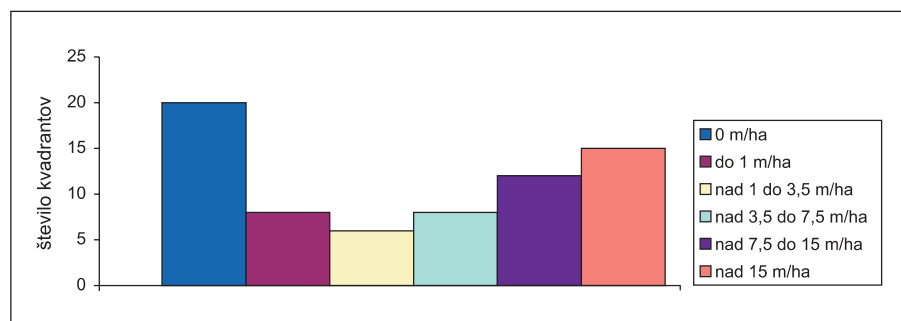
Grafikon 3: Pojavljanje muflonov glede na gostoto cestnega omrežja
