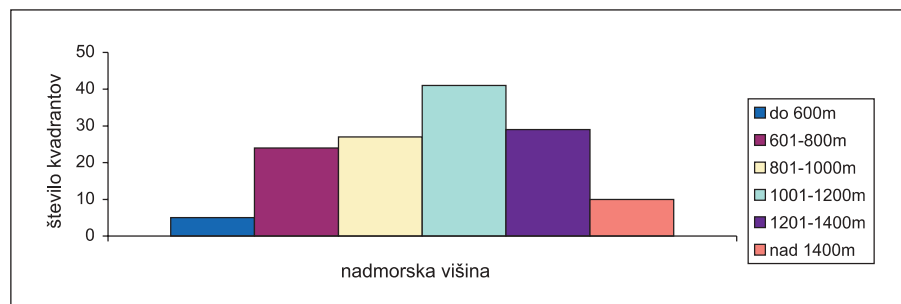
Grafikon 1: Pojavljanje muflonov glede na nadmorsko višino
