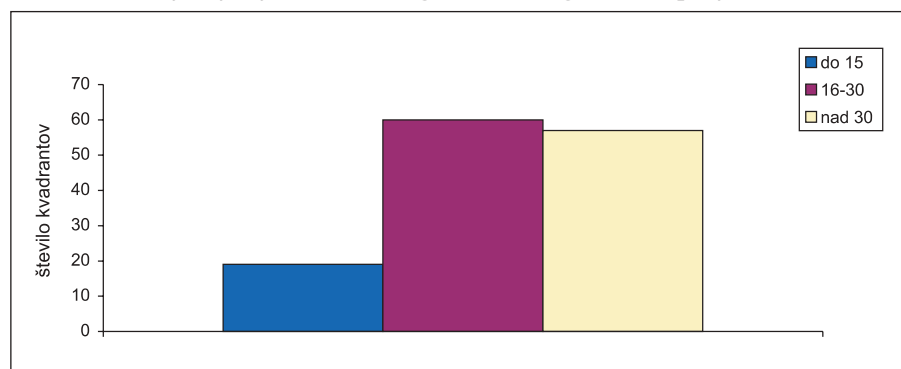
Grafikon 2: Pojavljanje muflonov glede na nagib (v stopinjah)
