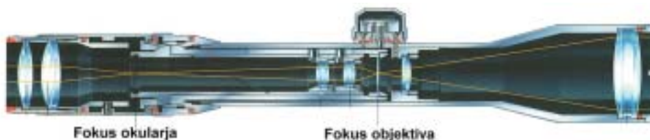
Lega goriščnih točk okularja in objektivna
