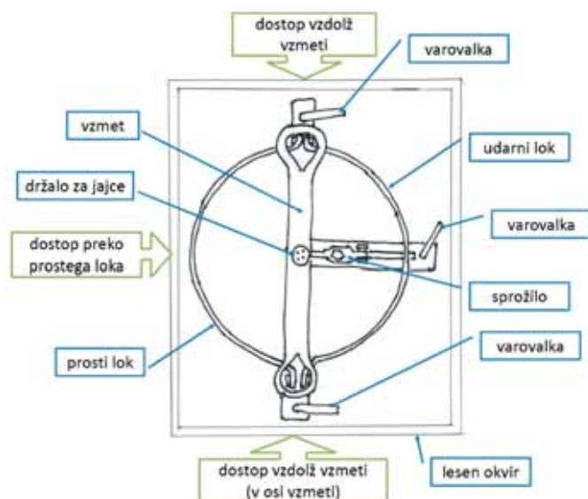
Skica dvigalke z dvema vzmetema
