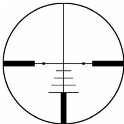
Slika 1: TDS-merilni križ, s katerim je opremljen strelni daljnogled Swarovski Habicht 4-16 x 50 PV. Pomožni piki (točki) sredinske niti merilnega križa (in oba kraja posameznih zastavic) sta namenjeni za merjenje na premikajoče se cilje oziroma za izravnavo vodoravnega odklona krogle zaradi učinka bočnega vetra, ko moramo pomeriti pred cilj. Štiri dodatne zastavice so namenjene za streljanje na daleč, na večje razdalje od 100 m, ko je treba pomeriti nad cilj.
