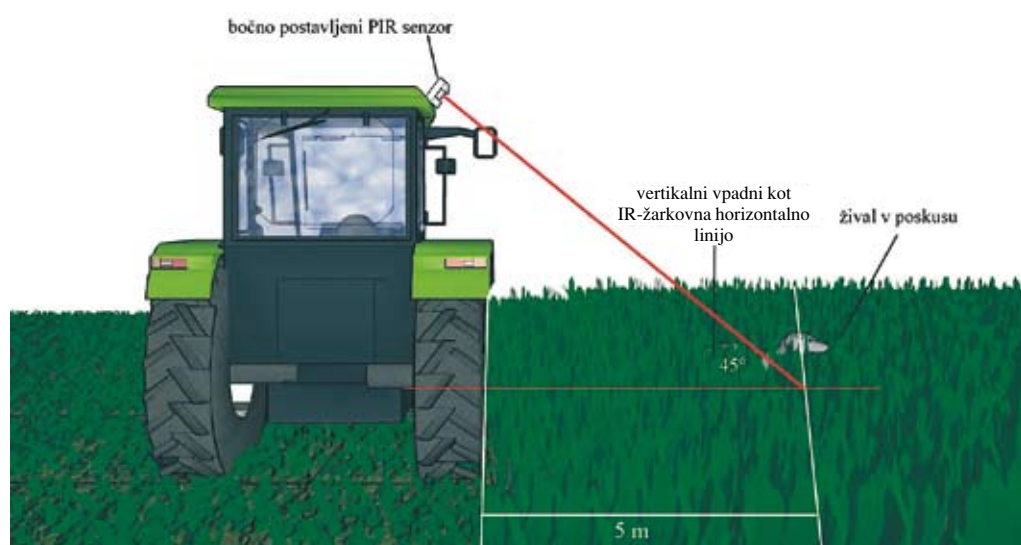
Slika 5: Prikaz odkrivanja živali z bočno namestitvijo IR-senzorjev
