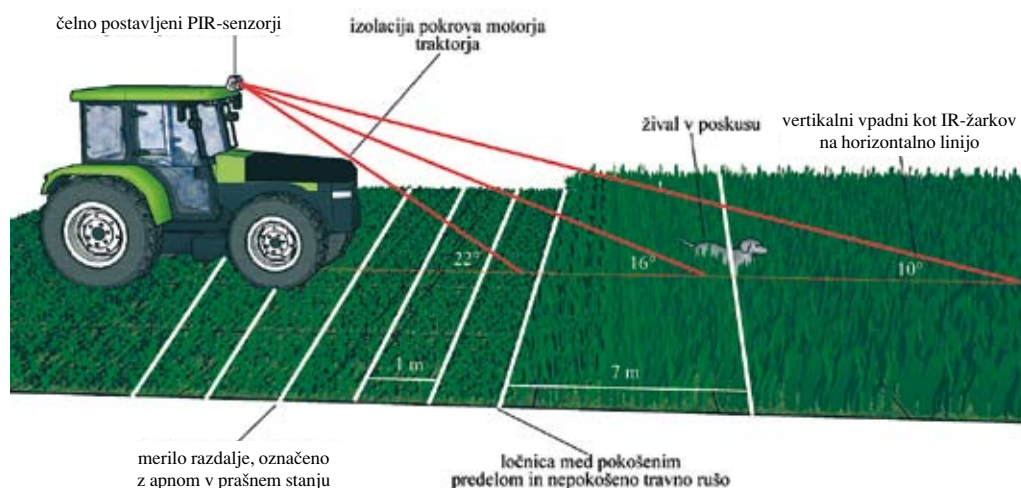
Slika 4: Prikaz odkrivanja živali s čelno namestitvijo IR-senzorjev
