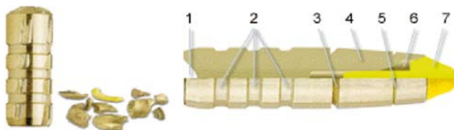
Slika 3: Razletavna krogla brez svinca. Zaradi razbitja prednjega dela povzroči delni šok. Primerna je za lažjo divjad. 1. balistična kalota, 2. razbremenilni žlebiči, 3. ostra zarez, 4. krušljiva trda medenina, 5. brazda, 6. polnitev
