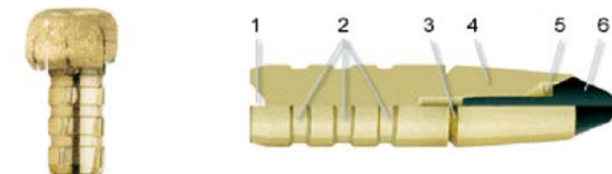
Slika 4: Deformacijska krogla brez svinca povzroči dober udarni val in zanesljiv izstrel. Primerna je za težjo divjad in dopolnjuje razletavno kroglo. 4. posebna, delno gnetljiva medenina.
