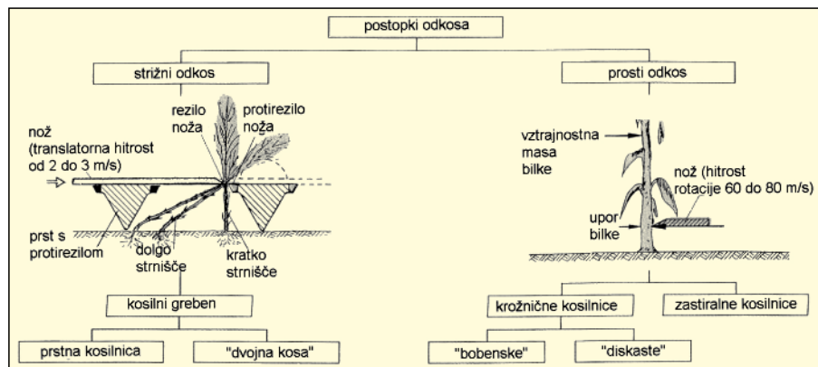
Slika 4: Načini odkosa pri kosilnicah
