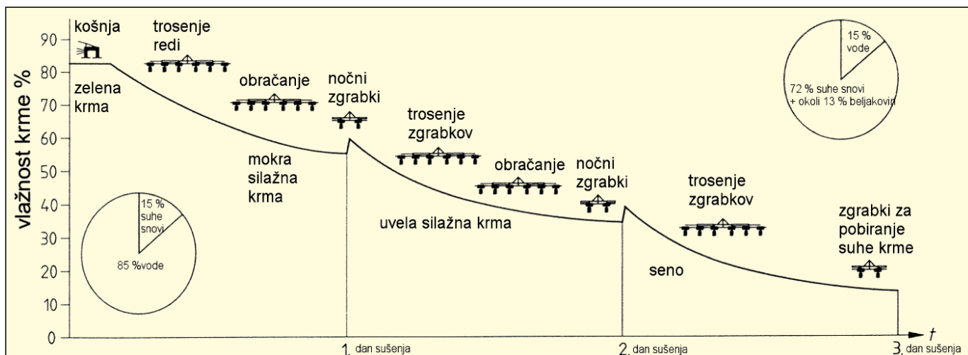
Slika 6: Postopek sušenja sena z dnevnimi opravili pri sušenju krme
