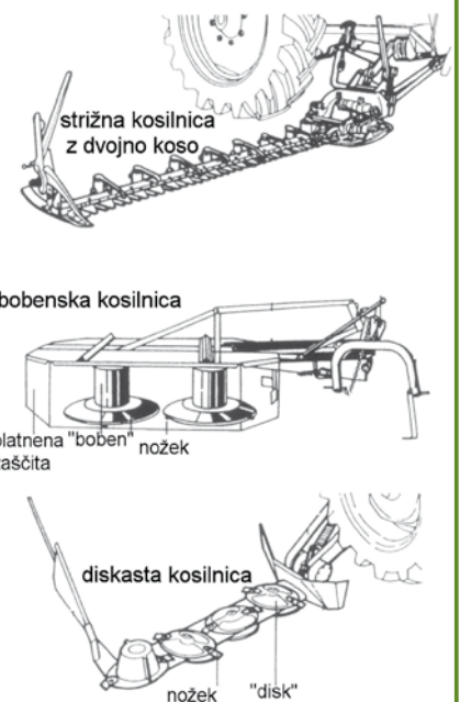
Slika 2: Izvedbe kosilnic
