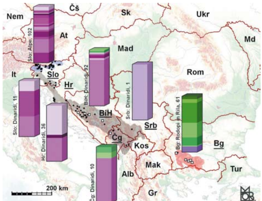
Slika 1: Zemljevid lokacij vzorčenja divjega petelina ( Tetrao urogallus ) na Balkanu in v slovenskih Alpah s stolpčnimi diagrami genetske sestave po vzorčenih državah in gorskih verigah. Slovenske Alpe so senčene modro, Dinaridi sivo, pogorje Rodopi – Rila – Pirin pa rdeče. S črnimi točkami so označene lokacije, kjer so odkrili zgolj predstavnike severne genetske linije, z belimi kvadrati s črno obrobo pa lokacije, kjer so odkrili tudi ali samo predstavnike južne genetske linije. Vsak izmed 30 unikatnih genotipov, ki so jih odkrili v tej raziskavi, je predstavljen v stolpcnem diagramu s svojo barvo: severna genetska linija z vijoličnimi, južna genetska linija z zelenimi odtenki. S slike je razvidna prevlada severne genetske linije v Alpah in Dinaridih, prisotnost južne genetske linije v osrednjih in JV Dinaridih ter prevlada le-te v pogorju Rodopov in Rile. Prav tako je razvidna velika genotipska raznolikost slovenske alpske populacije, ki je največja od vseh treh populacij, analiziranih v tej raziskavi. Ob vsakem stolpcnem diagramu je zabeleženo: okrajšava države, gorovje in število analiziranih vzorcev. Alb: Albanija, At: Avstrija, BiH: Bosna in Hercegovina, Bg: Bolgarija, Čg: Črna gora, Čs: Češka, Gr: Grčija, Hr: Hrvaška, It: Italija, Kos: Kosovo, Mad: Madžarska, Mak: Makedonija, Md: Moldavija, Nem: Nemčija, Rom: Romunija, Sk: Slovaška, Slo: Slovenija, Srb: Srbija, Tur: Turčija, Ukr: Ukrajina. Okrajšave vzorčenih držav so podčrtane. (Grafika: Marko Bajc)
