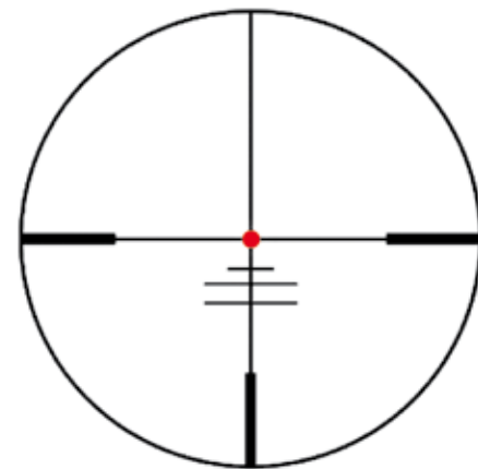
Slika 6: Balistični merilni križ 4A-300 tovarne Swarovski, ki ga vgrajuje v nekatere modele strelnih daljnogledov.
