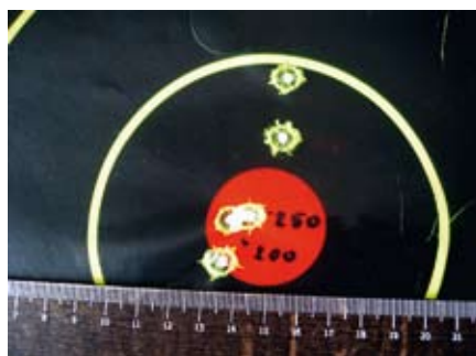
Slika 12. Na razdalji 200 m zadeva puška v piko brez višinskih popravkov, ker je pristreljena na UPR (leva dva zadetka v rdeč center tarče). Z ustreznim popravkom na balističnem bobniču strelnega daljnogleda Swarovski je zadel strel v piko (skrajni desni zadetek v sredino tarče – center). Zgornja zadetka na razdalji 300 m sta po višini razmaknjena za 2,1 cm (nastavitev 300 m na balističnem bobniču). Z natančno puško v razantnem kalibru 8 x 68 S je torej mogoče zanesljivo streljati in natančno zadevati cilje na lovske »pravičnih razdaljah« in po potrebi še precej večjih.
