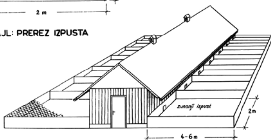
Načrt jerebičarne, ki so ga pripravili strokovnjaki lovskega oddelka Gozdarskega inštituta.
