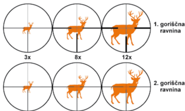
Slika 3: V zgornji vrsti je prikazano spreminjanje velikosti namerilnega križa s spreminjanjem povečave strelnega daljnogleda. Križ se namreč v takšnih strelnih daljnogledih povečuje skupaj z opazovano tarčo in pri vseh povečavah zakriva enako velik del tarče. V strelnih daljnogledih, ki imajo namerilni križ nameščen v drugi goriščni ravnini, se le-ta z večanjem povečave daljnogleda na tarči krči. Pri največji povečavi tako pokriva zelo majhen del tarče.
