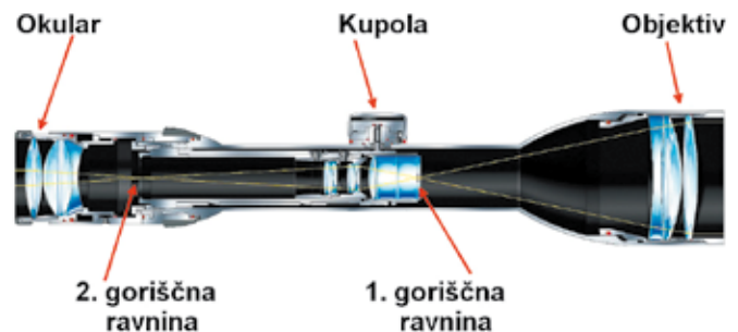
Slika 2: Osnovni sklopi vsakega strelnega daljnogleda so objektiv, okular, kupole za nastavitve pozicije namerilnega križa ter obe goriščni ravni, v katerih je lahko nameščen namerilni križ.
