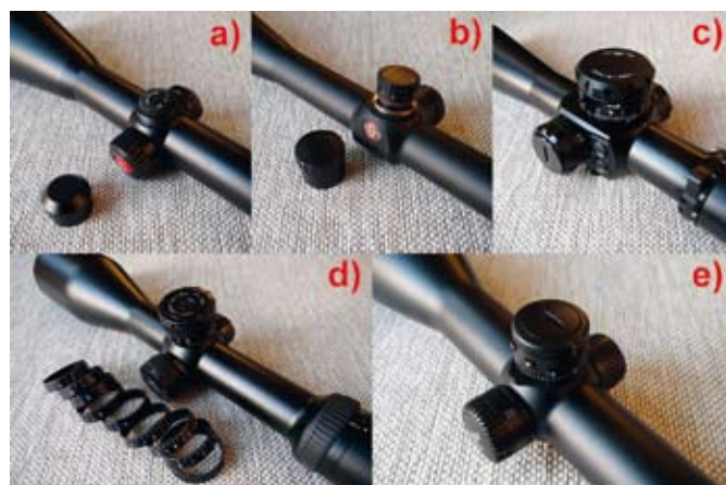
Slika 4: V zgornji vrsti so prikazni tipi kupol na strelnih daljnogledih, in sicer: a) pokrite, b) športne in c) taktične. V spodnji vrsti sta prikazana oba tipa lovskih balističnih kupol, in sicer d) z zamenljivimi obroči z oznakami in e) z nastavljljivimi razdelki.
