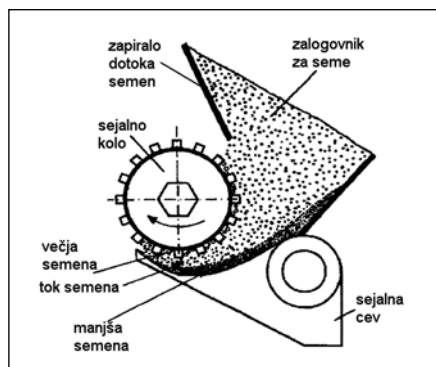
Slika 5 b: Odgrebala pri pnevmatični sejalnici
