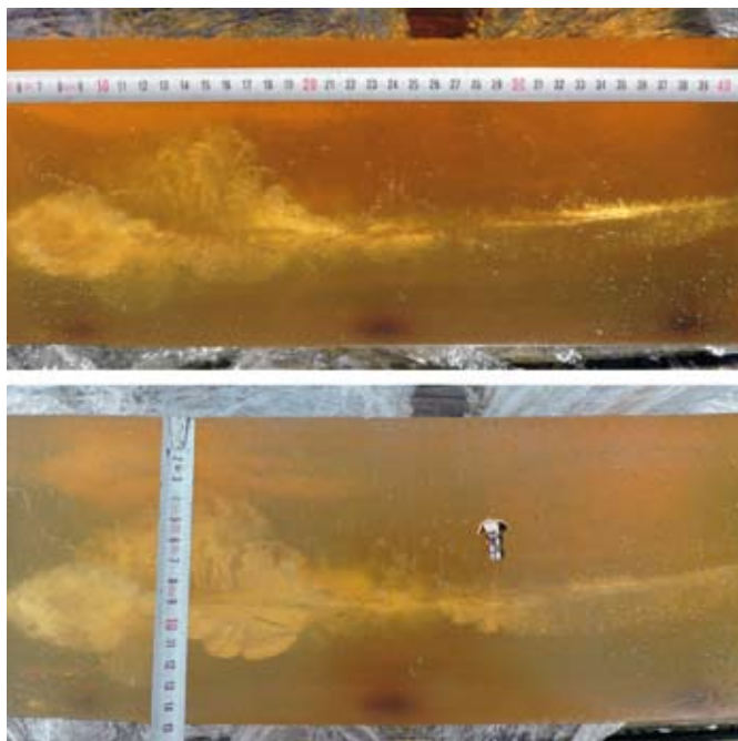
10. Strelni kanal v balistični želatini
