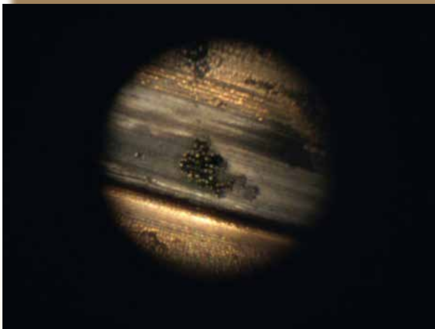
Slika 2: Notranjost cevi starejše risanice 6,5 x 68
