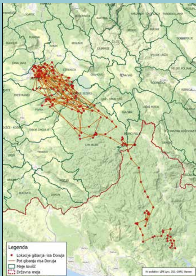
Slika 4: Zemljevid poti gibanja risa Doruja od izpusta do ustalitve na novo ustvarjenem teritoriju
