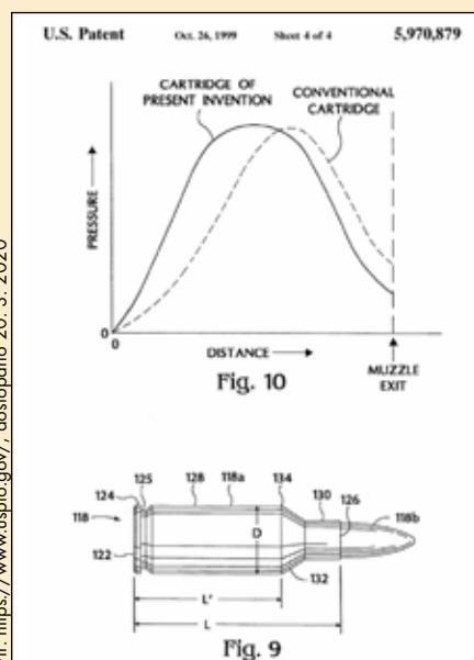
Slika 4: Izsek iz patenta Ricka Jamisona
