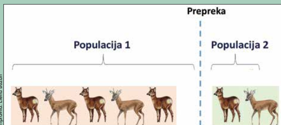
Slika 2: Naravne ali antropogene prepreke lahko prekinajo genski pretok znotraj populacije, zato se osebki in novonastale delne populacije čez čas začno razlikovati v genetskih značilnostih.
