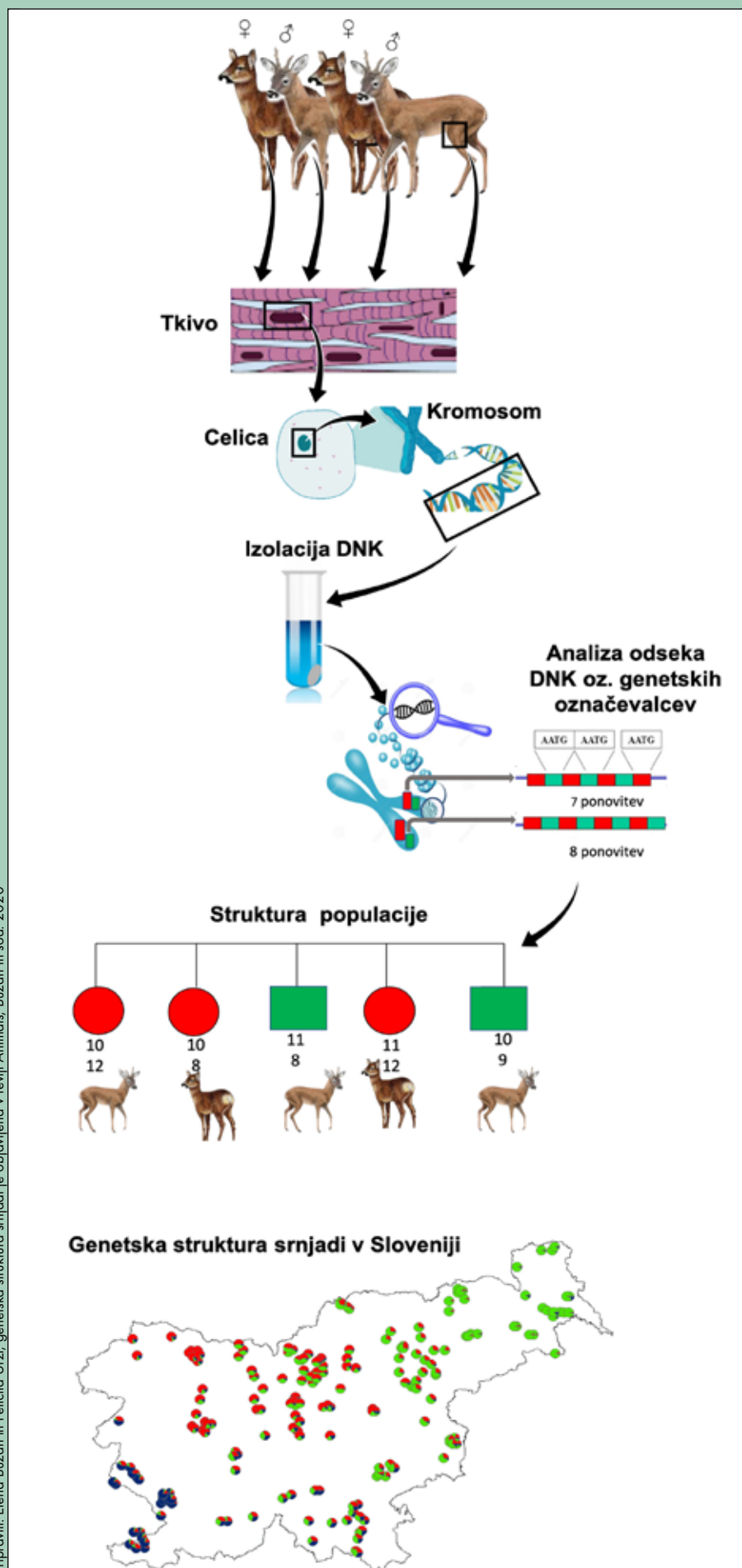
Slika 3: Shematski prikaz poteka genetske analize na primeru srnjadi v Sloveniji: odvzem tkiva, izolacija DNK, analiza molekularnih označevalcev (vsak osebek ima svojo »molekulsko (genetsko) kodo«) in prostorski prikaz razlik v genetski strukturi ciljne vrste
