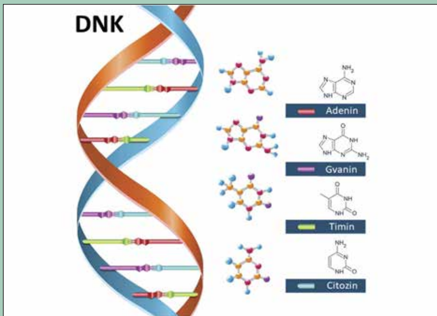
Slika 1: Dvojna vijačnica molekule DNK. Razvidni so osnovni gradniki (nukleotidi) in povezljiva (komplementarna) dela, kjer se gradniki povezujejo in tvorijo značilno dvojno-vijačno strukturo.
