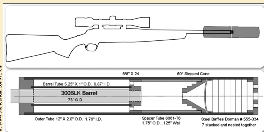
Slika 6: Shema namestitve dušilca zvoka, ki ga namestimo nazaj prek ustja cevi.
