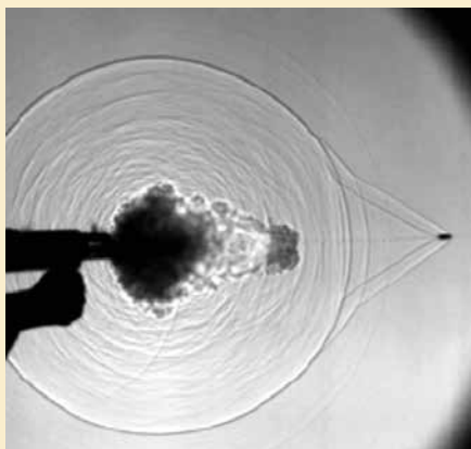
Slika 3: Udarni val ob strelu kalibra 7,62 x 39
