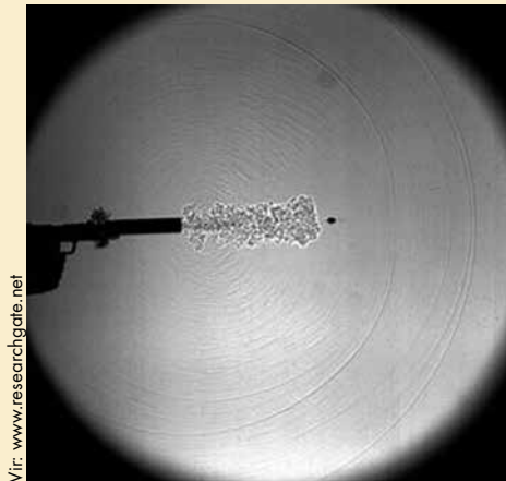
Slika 4: Udarni val ob strelu kalibra .45 ACP brez dušilca zvoka in z nameščenim dušilcem zvoka
