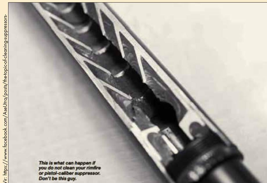
Prikaz notranjosti dušilca poka Ase-Utra, prva komora, prerez
