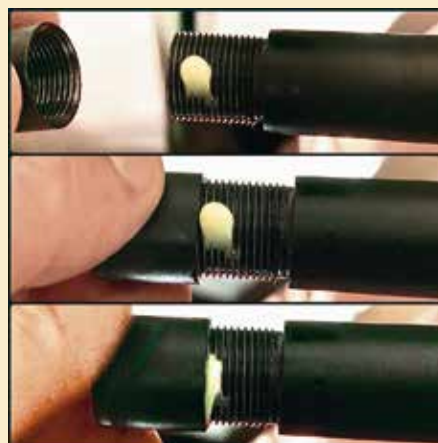
Mazanje navojev na ustju cevi z mastjo
