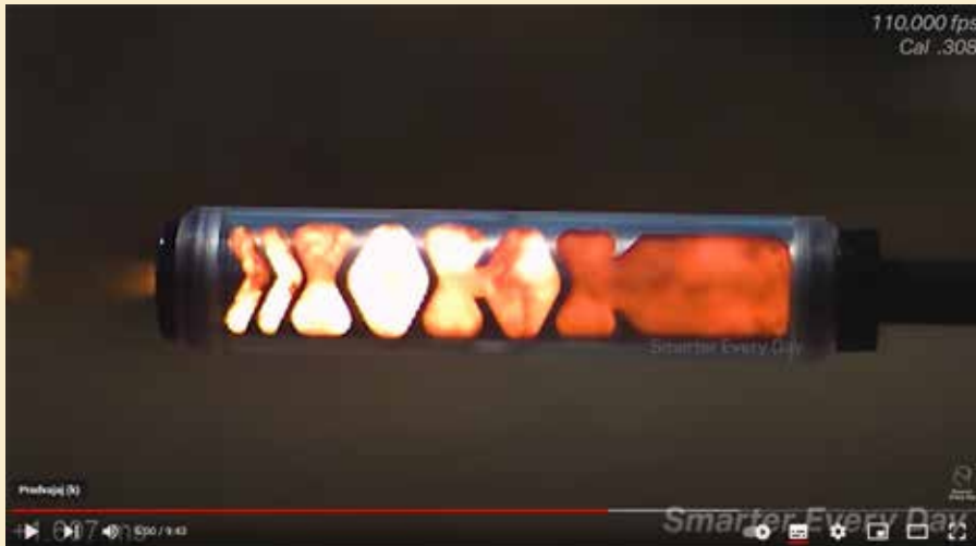
Notranjost dušilca poka ob strelu
